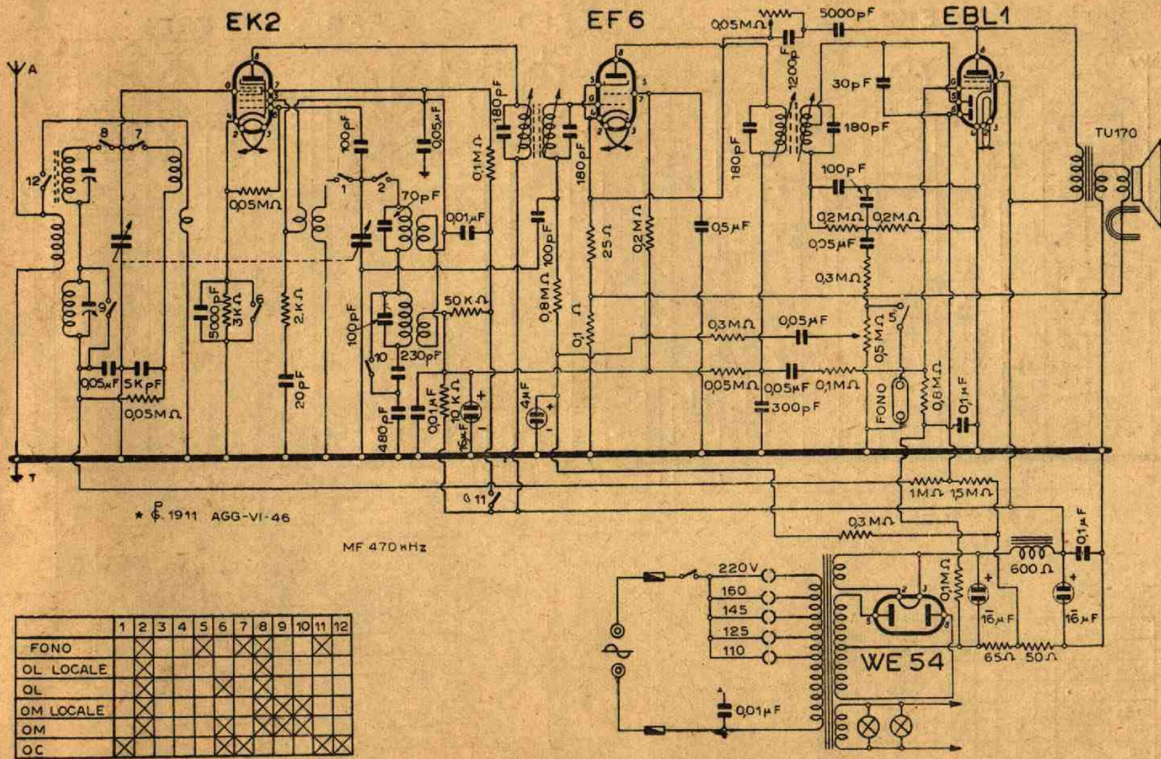
Lo schema elettrico del Mod. 384 Minerva
